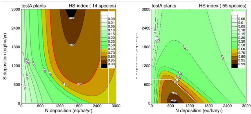
Figure IT-3. Site IT08.
