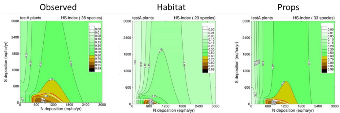
Figure IT-1. Site IT05.
